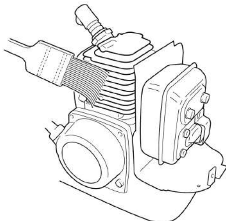
Рис. 21 Очистка рёбер охлаждения цилиндра
