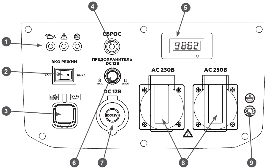
Рис. 5. Панель управления
