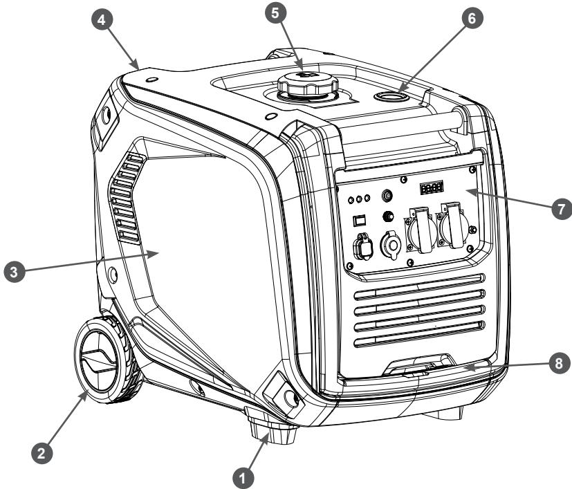
Рис. 1. Основные узлы и органы управления (вид спереди)
