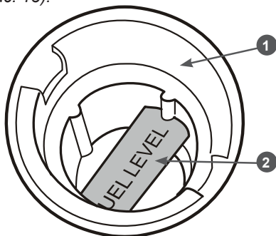
Рис. 13. Указатель максимального уровня топлива в топливном баке
