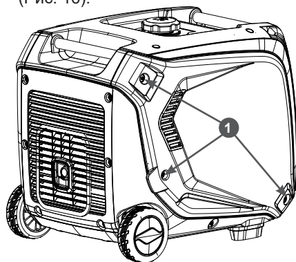
Рис. 16. Снятие левой панели корпуса
