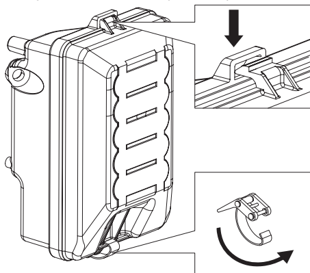
Рис. 19. Снятие крышки воздушного фильтра
