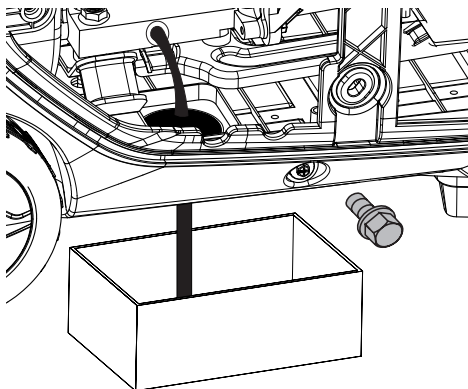
Рис. 18. Слив масла с картера двигателя
