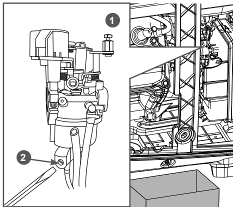
Рис. 21. Слив топлива из карбюратора
