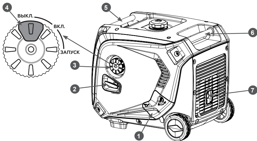
Рис. 2. Основные узлы и органы управления (вид сзади)
