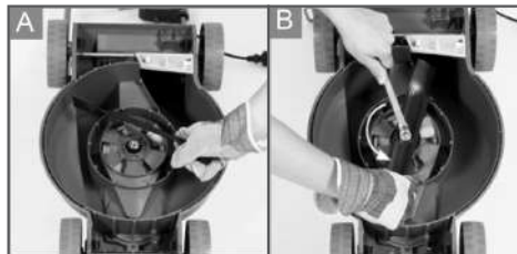
Рис.5 Установка ножа
