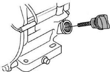
Рис. 21. Крышка-щуп нижней маслозаливной горловины
