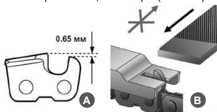
Рис. 39 Проверка высоты ограничителя глубины резания
