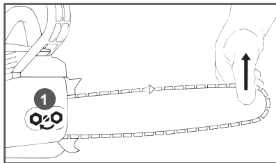
Рис. 6. Натяжение цепи
