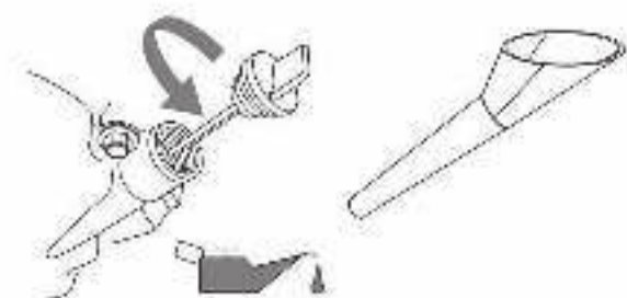
Рисунок 4-1. Заливка моторного масла
