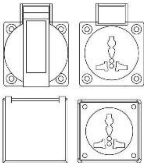
Рисунок 2-3. Розетка переменного тока
