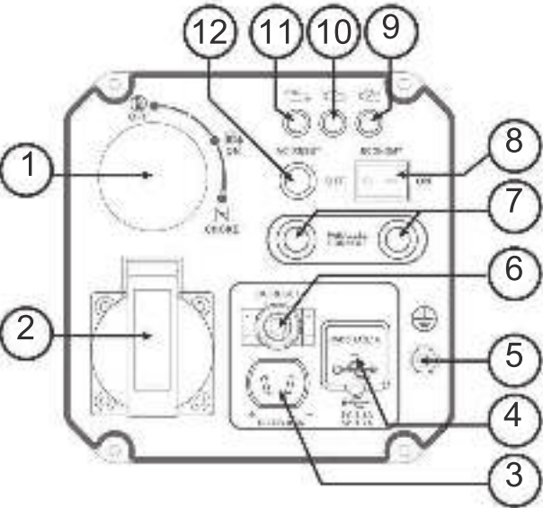
Рисунок 2-2. Панель управления
