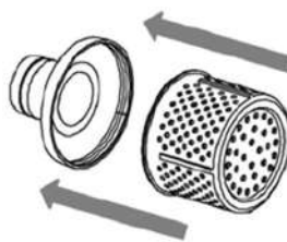
Рис. 9 Сборка всасывающего фильтра
