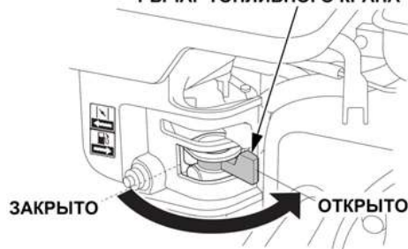
Рис. 14 Рычаг топливного крана
