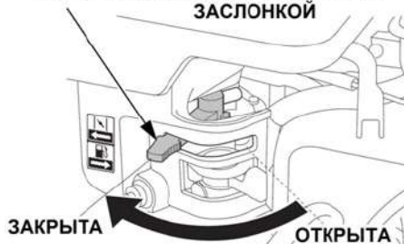
Рис. 14 Рычаг управления воздушной заслонкой
