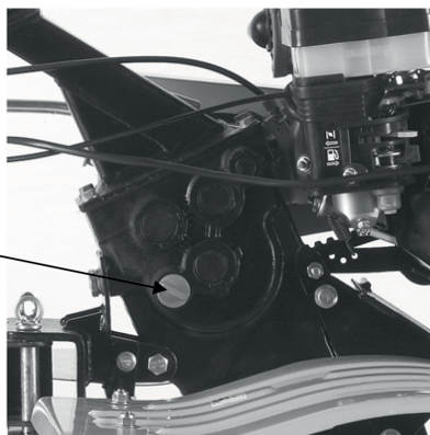
Пробка маслозаливной горловины редуктора
