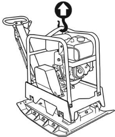
Рис. 30 Точка зацепа крюка подъемного устройства
