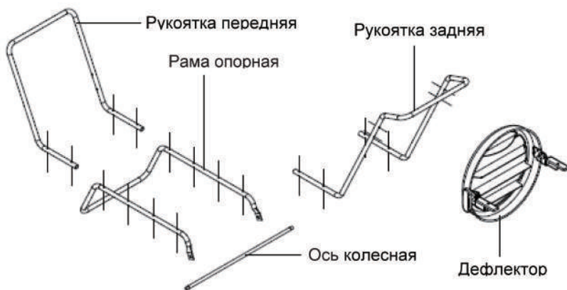
Рис 3. Рама опорная
