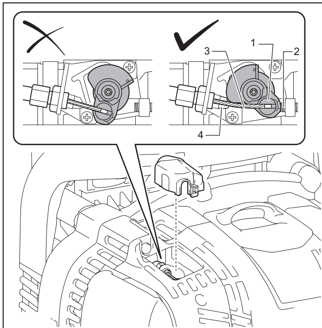
► 1. Reglerventil 2. Justerskruv, tomgång 3. Styrkabel 4. Plugg, reglerventil
