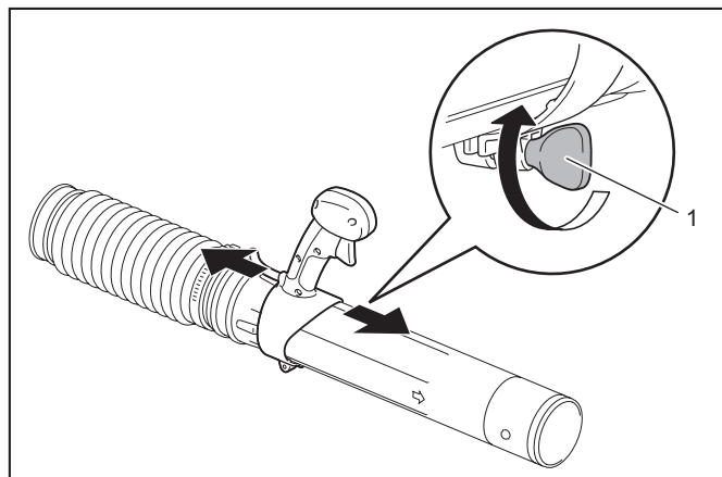
► 1. Skruv
