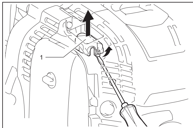
► 1. Крышка карбюратора
