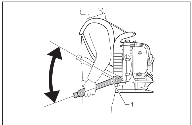
► 1. Kontrollarm
