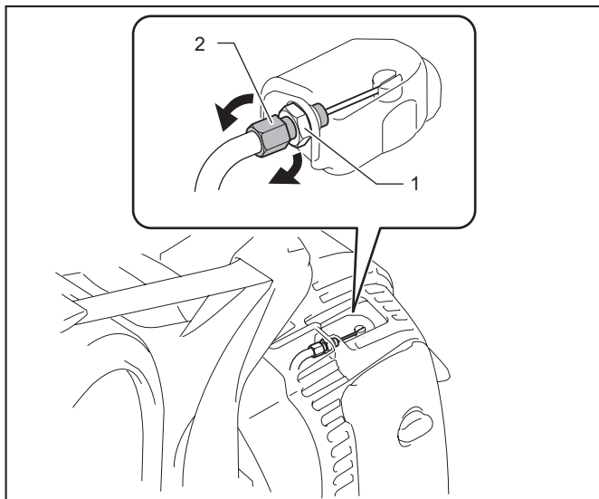
► 1. Låsmutter 2. Justerbult, kabel
