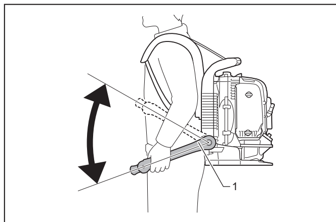
► 1. Styrarm
