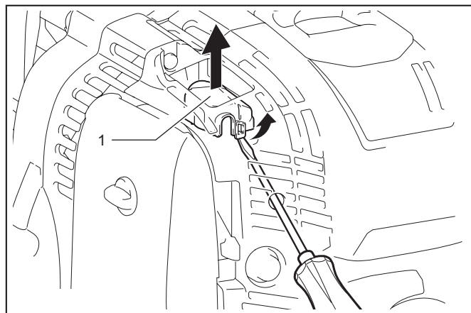
► 1. Förgasarkåpa
