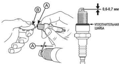
Рис. 13 Проверка зазора между электродами
