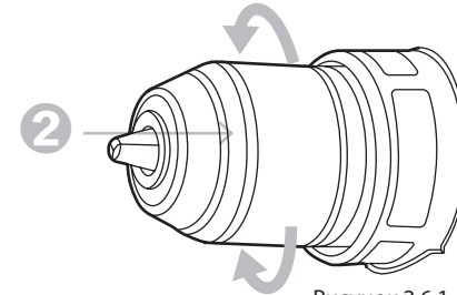
Рисунок 2.6.1. Установка оснастки
