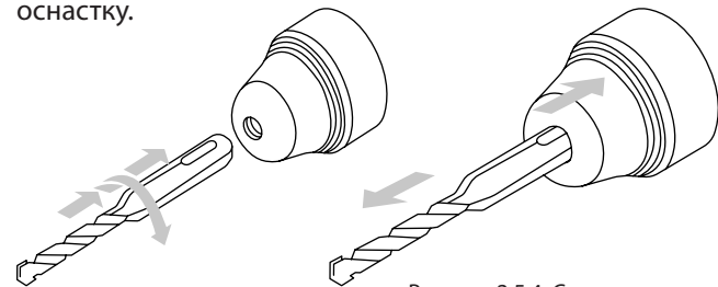
Рисунок 2.5.4. Снятие оснастки
