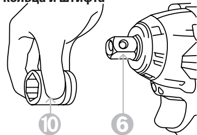
Рисунок 2.3.2. Установка головки
