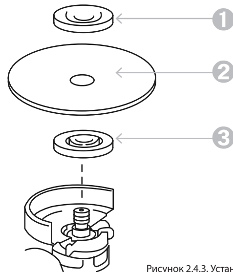
Рисунок 2.4.3. Установка оснастки
