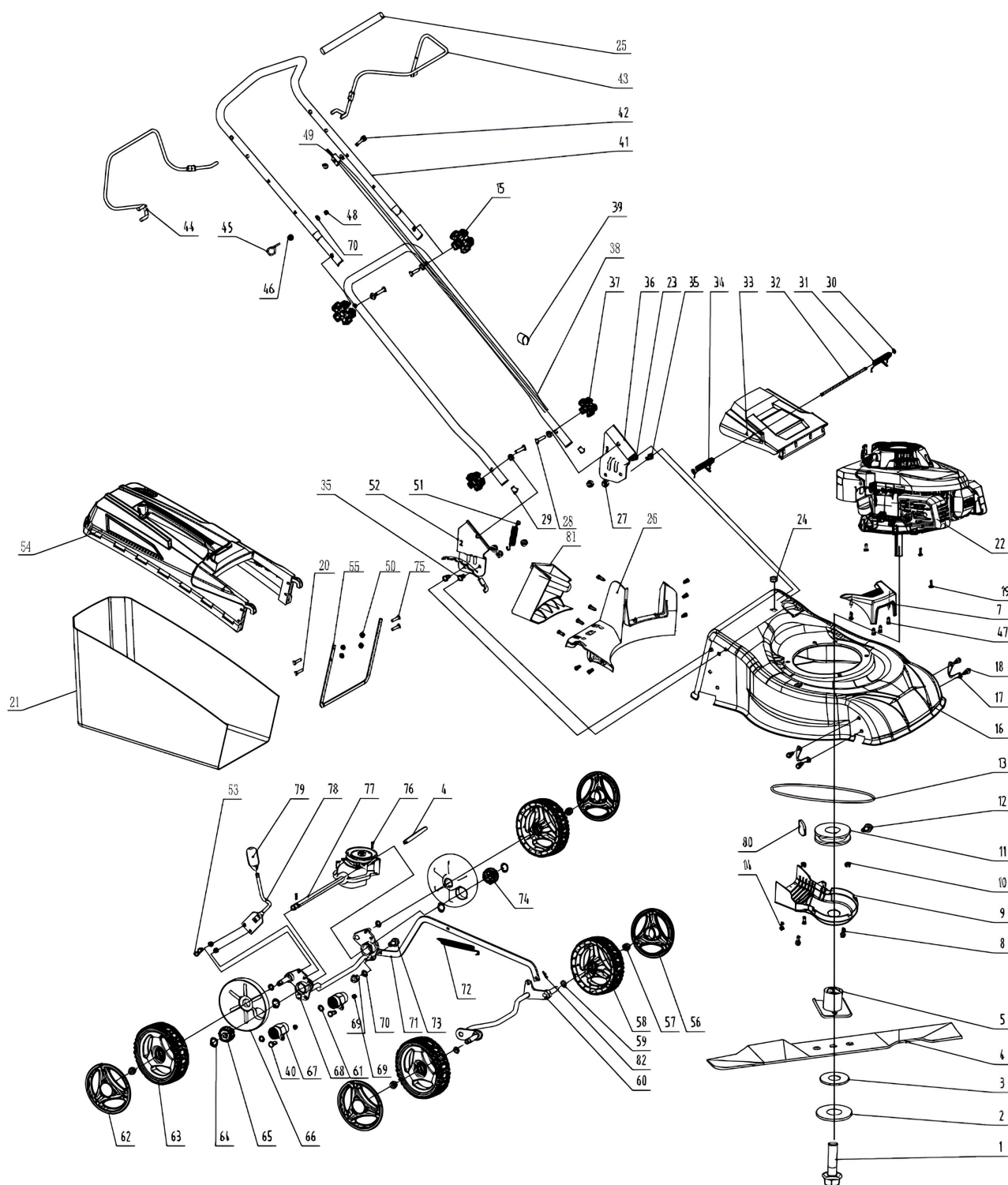
РИСУНОК А. ГАЗОНОКОСИЛКА В РАЗБОРЕ
