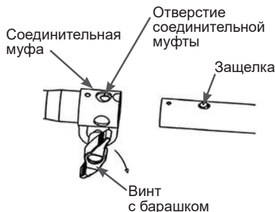
Рис. 5 Установка нижней штанги
