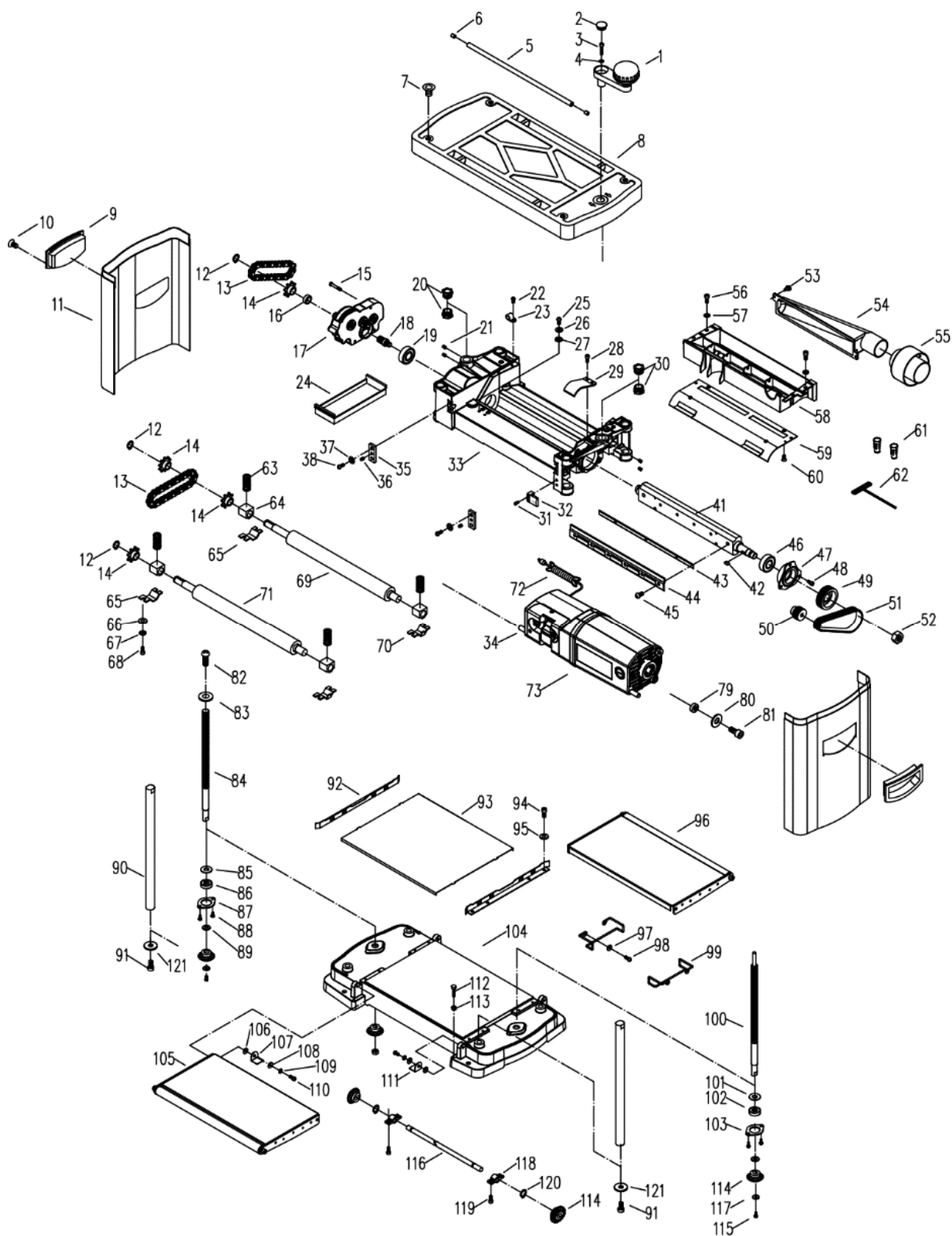
Рисунок 14. Взрыв-схема для модели BELMASH P1800
