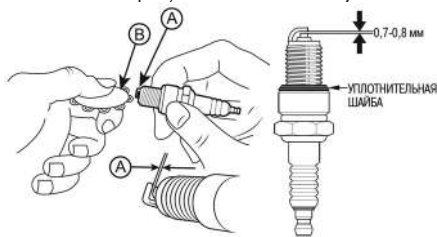
Рис. 19. Проверка зазора между электродами
