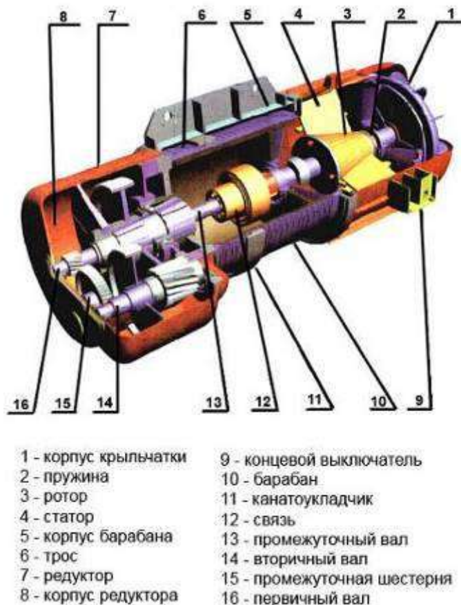
Рисунок 1. Электротельфер типа MD (разрез)
