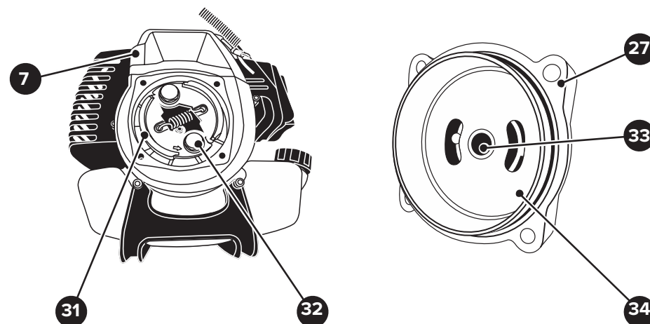
7. Двигатель 31. Корпус (узел сцепления) 32. Кулачки (2 шт.)
