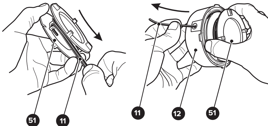
11. Режущий корд 12. Режущая головка
