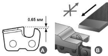
Рис. 20 Проверка высоты ограничителя глубины резания
