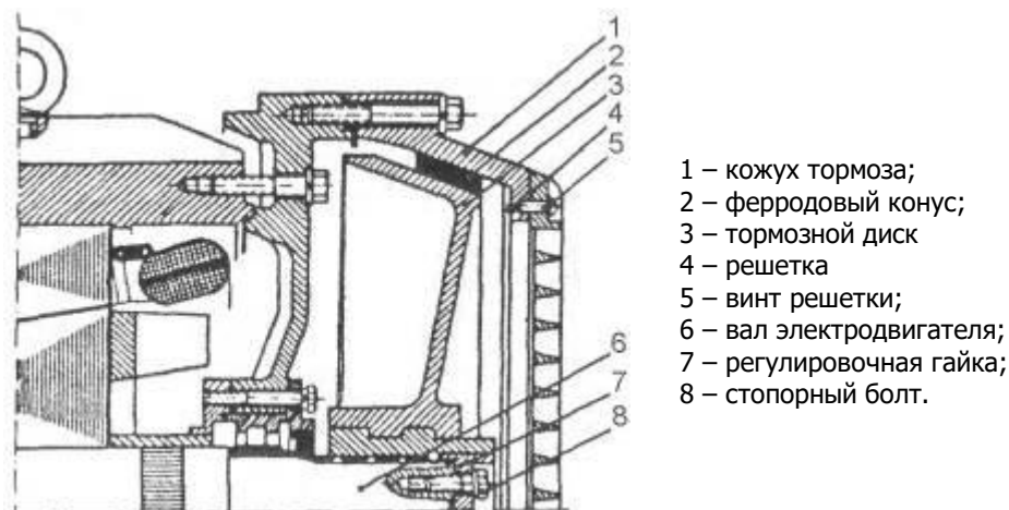
Рисунок 18. Частичный разрез электродвигателя подъемного механизма.
