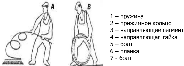
Рисунок 6. Канатоукладчик – развернутый вид.
