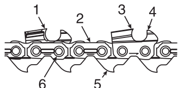
Рис. 15 Конструкция пильной цепи
