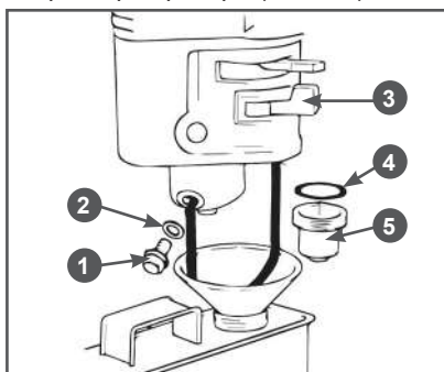
Рис. 20 Обслуживание фильтра-отстойника
