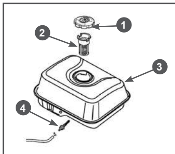
Рис. 18 Топливные фильтры
