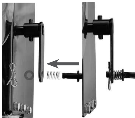
Рис. 14 Подключение троса к нижнему рычагу
