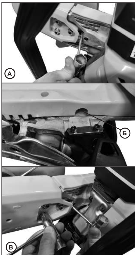
Рис. 24 Натяжение ремня в положении режущего узла снаружи
