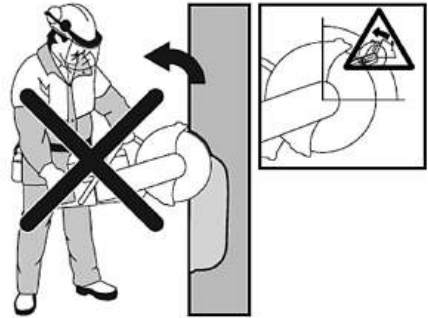
Рис. 14 Отдача вверх
