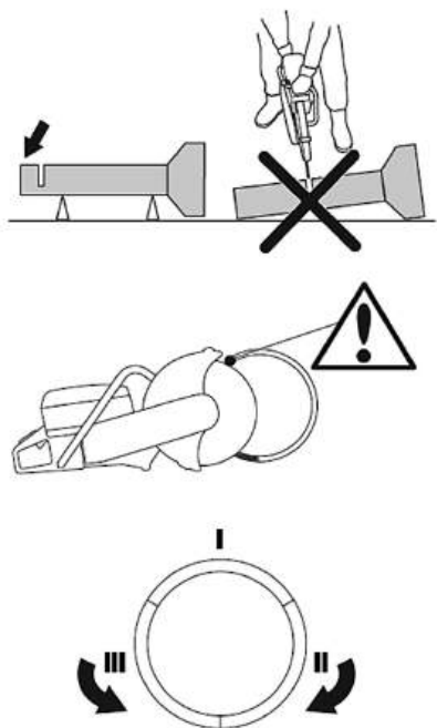
Рис. 16 Резка труб
