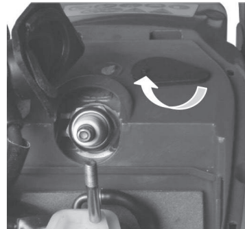
Փեղկի դիրքը «ամառ»
