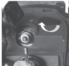
Положение заслонки «лето»
