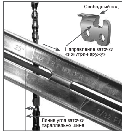
Рис. 37. Определение угла заточки
