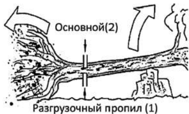
Рис. 26. Распиливание дерева, когда толстый ствол с комлевой частью находится под напряжением
