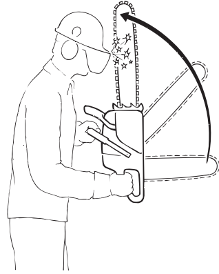
Рис.17. Отскок бензопилы
