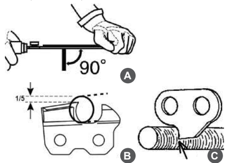
Рис. 38. Положение напильника при заточке
