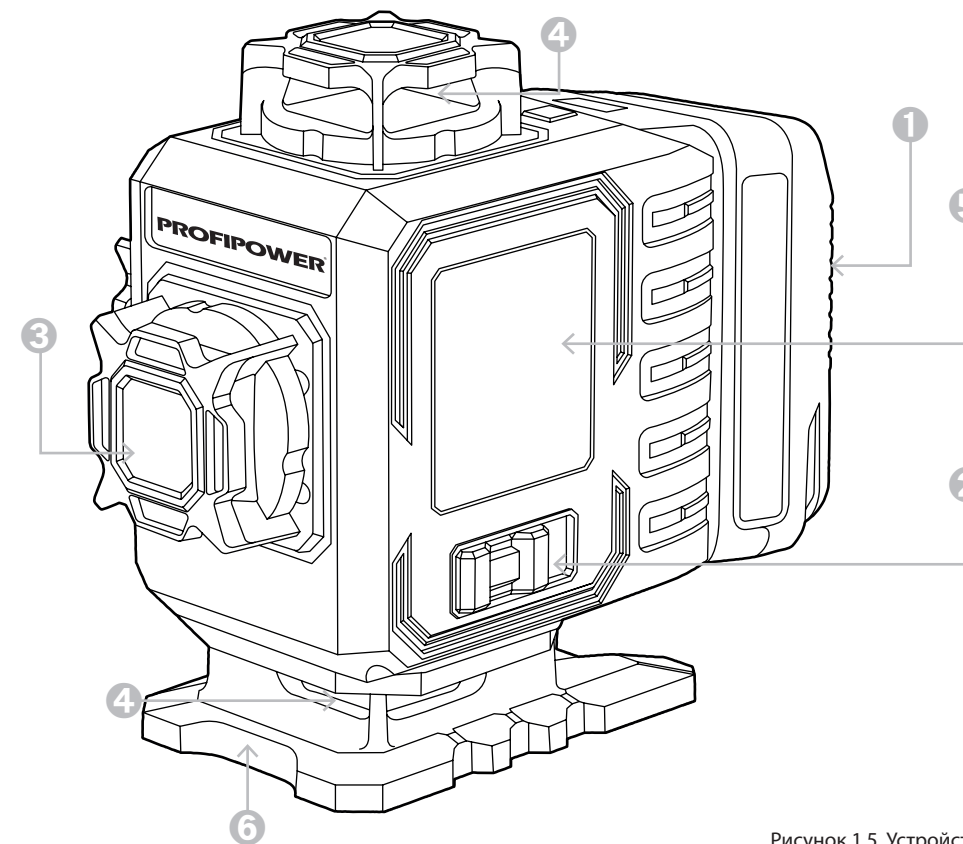
Рисунок 1.5. Устройство инструмента
