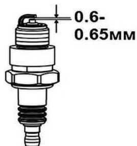
Рис. 23 Свеча зажигания
