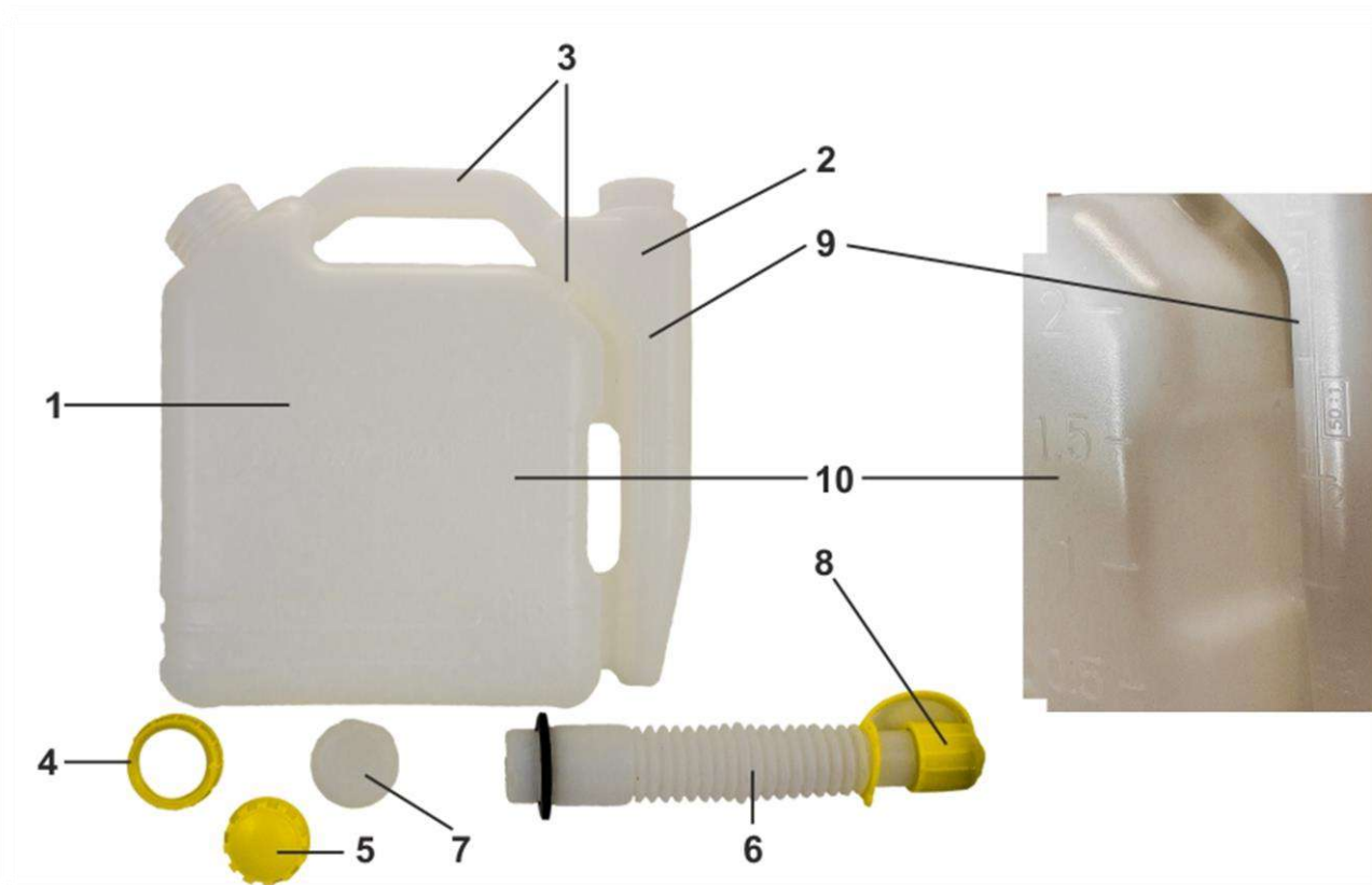
Рис. 1 Емкость для приготовления топливной смеси
