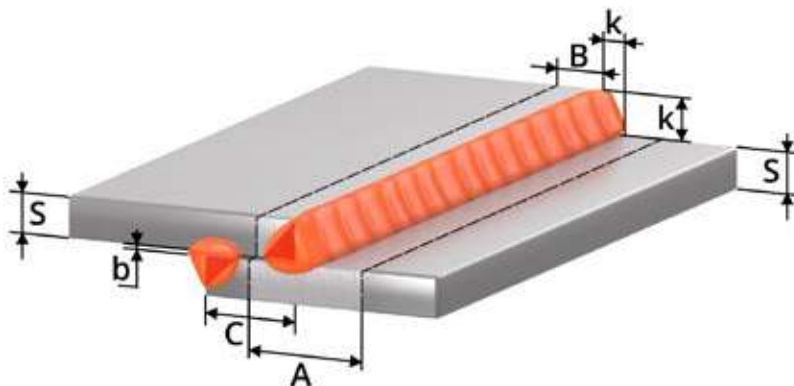
Рис. 13.0.5. Пример нахлесточного соединения.
