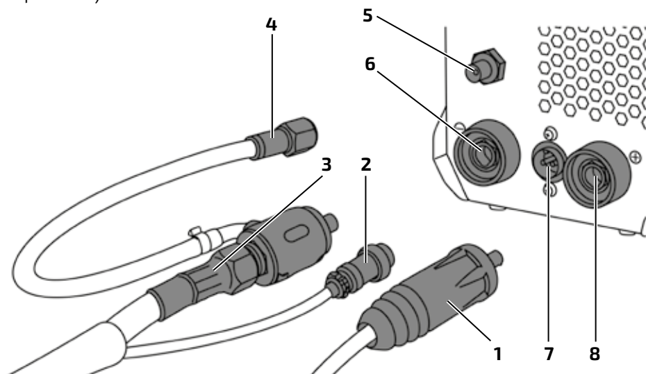
Рис. 8.0.3. Подключение.
