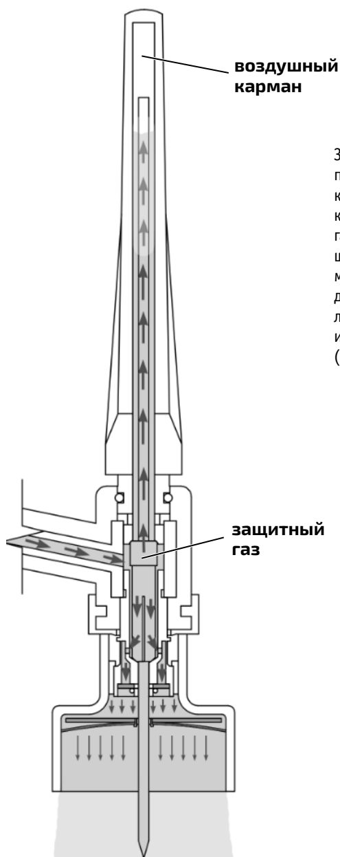
Рис. 9.7.2. Воздушный карман.
