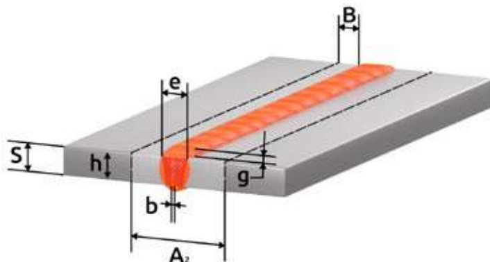
Рис. 13.0.1. Пример стыкового соединения.
