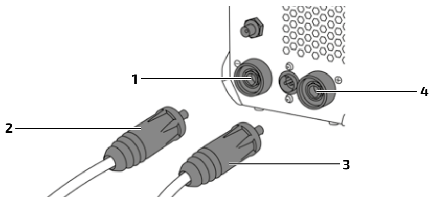
Рис. 10.0.2. Подключение в режиме MMA.
