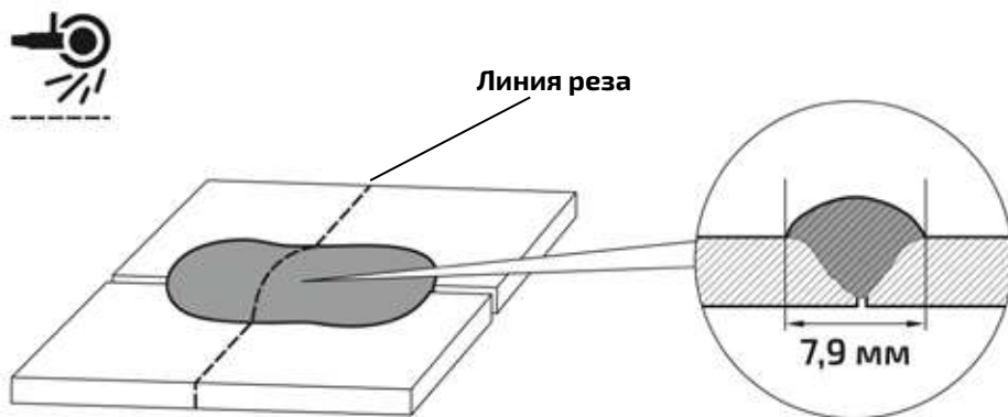
Рис. 12.2.1. Макрошлиф.
