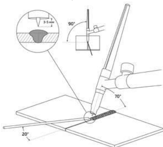
Рис. 9.9.1. Стыковое соединение.
