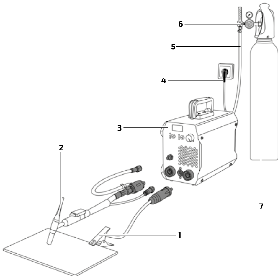
Рис. 8.0.1. Схема подключения оборудования с горелкой воздушного охлаждения.
