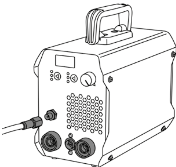
Рис. 8.0.2. Подключение защитного газа.
