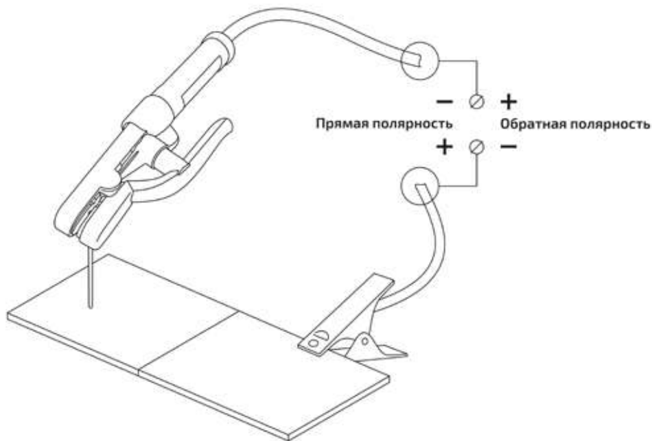
Рис. 11.2.1. Способы подключения.
