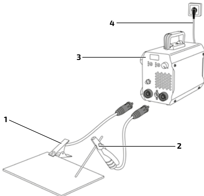
Рис. 10.0.1. Схема подключения оборудования.
