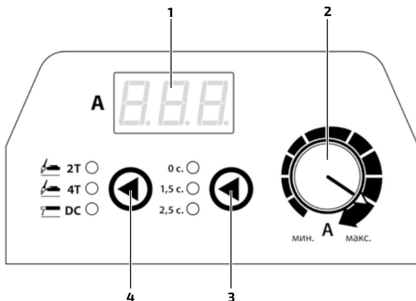
Рис. 7.0.1. Панель управления.
