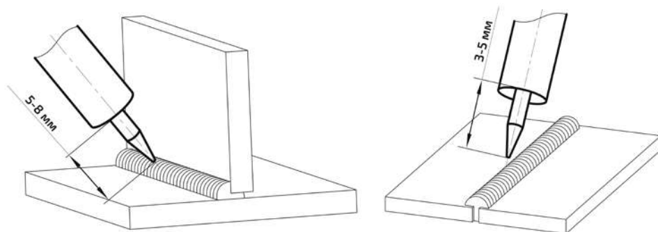
Рис. 9.5.1. Выпуск электрода.
