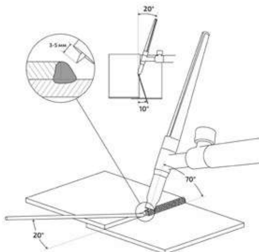
Рис. 9.9.2. Нахлесточное соединение.
