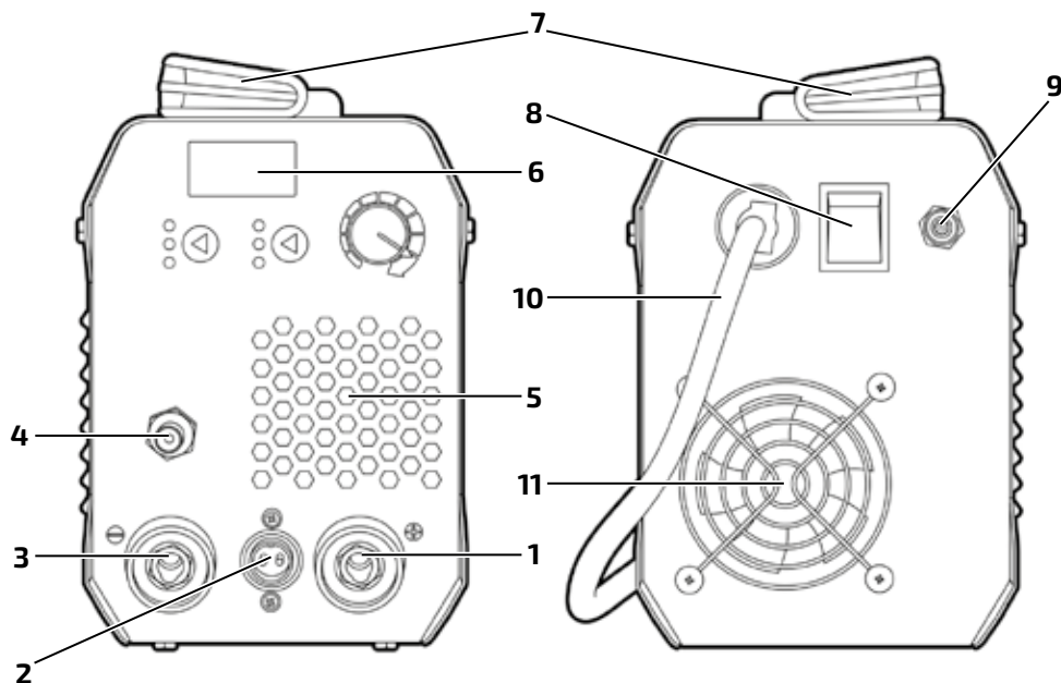
Рис. 6.0.1. Вид аппарата сзади и спереди.
