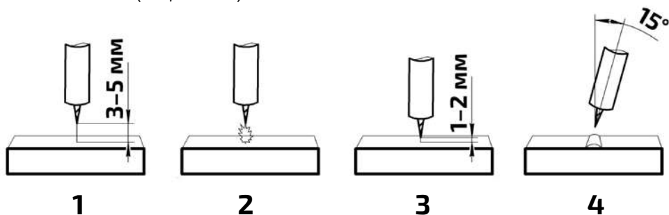
Рис.7.1.1. Высокочастотный поджиг дуги.
